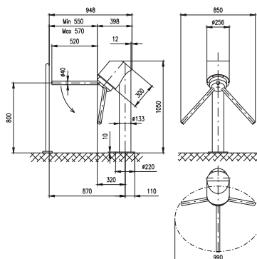
BAR-SKR-DropArm
